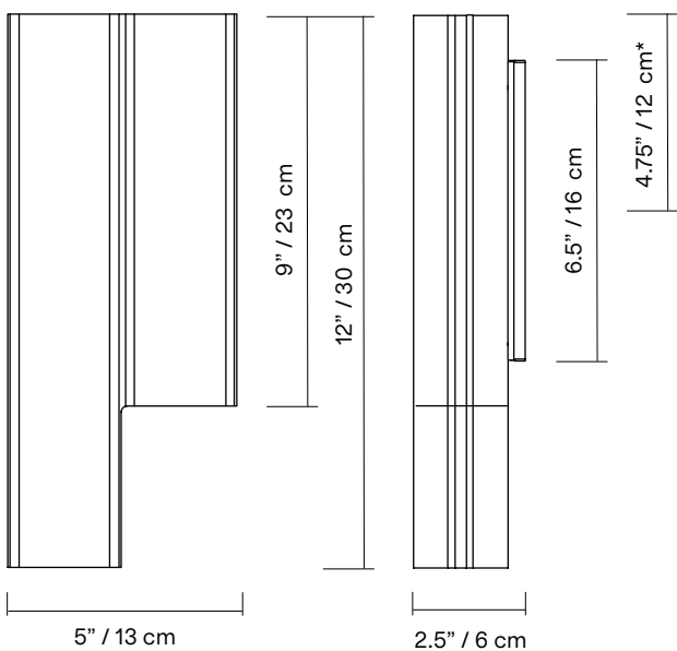
SILO 2WC
