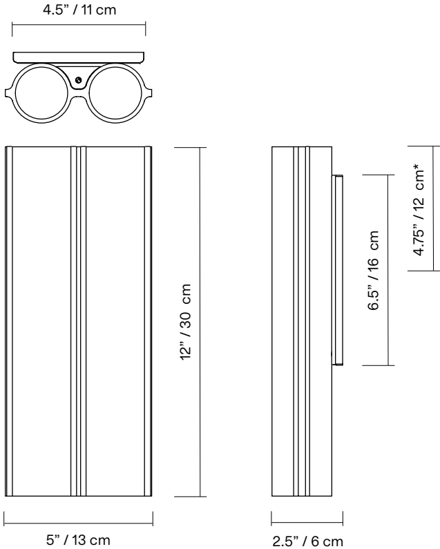
SILO 2WA
