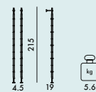
8933 2 struts
